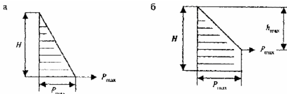
Рисунок 16.1 Расчетные эпюры бокового давления бетонной смеси а - гидростатическое давление; б - расчетное давление при уплотнении смеси внутренними вибраторами
