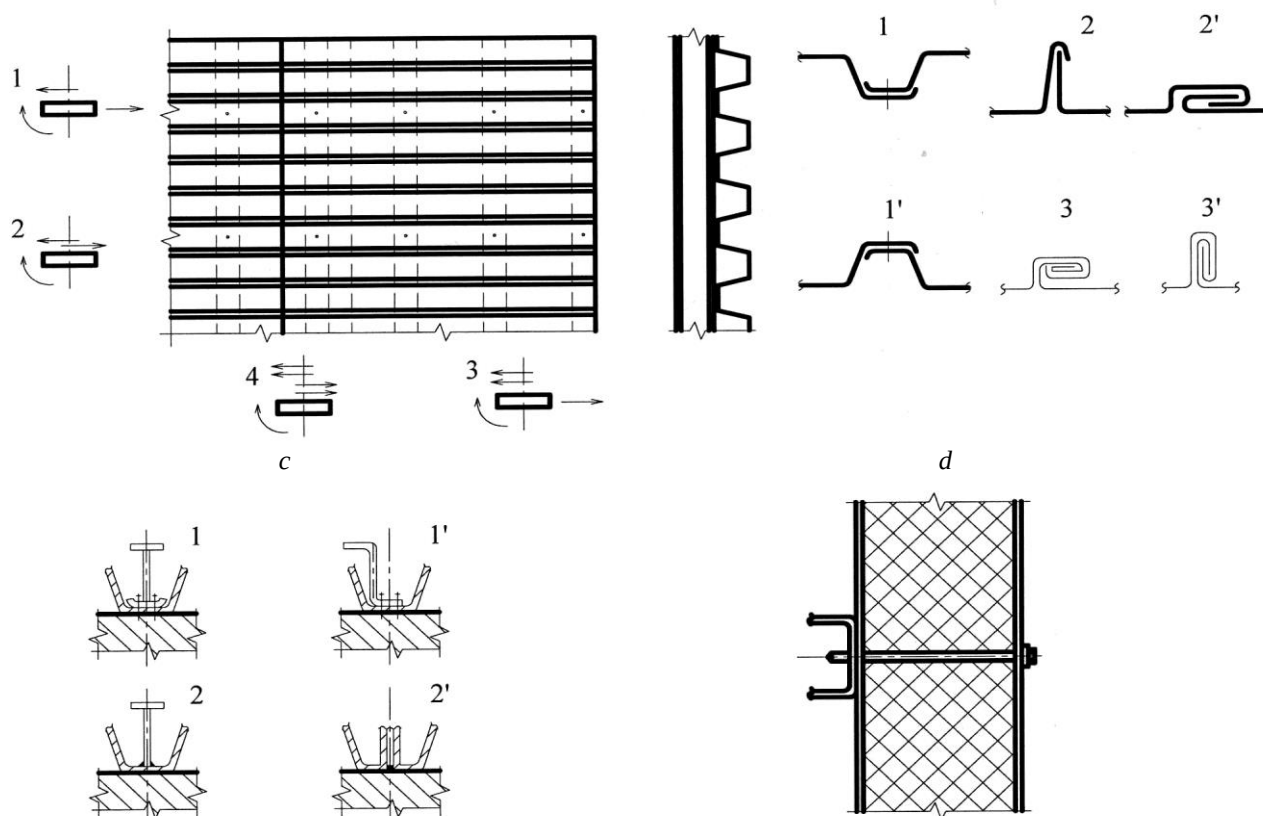
a – фрагмент конструкции покрытия со стальным профилированным настилом и схема действия сил на опорах (1- соединения в среднем участке; 2 и 3- соединения соответственно по продольным и поперечным полкам; 4 - соединения в месте пересечения продольных и поперечных полкам); b – схема соединений по продольным полкам (1 и 1' – при расположении полки внахлест в нижнем и верхнем положениях соответственно для утепленных и холодных покрытий; 2 и 2' – простой стоячий и лежащий фальцы; 3 и 3' – двойной фальц, стоячий и лежащий); c – сдвигустойчивые элементы (1 и 1' – на высокопрочных дюбелях; 2-на контактной сварке; 2'- на дуговой сварке); d – фрагмент трехслойной стеновой панели на самосверлящем винте
