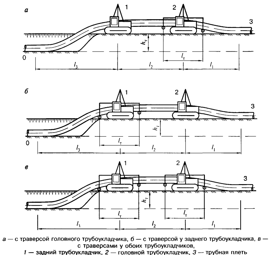
Рисунок 19 — Схемы укладки газопроводов с бермы траншеи с применением траверс
