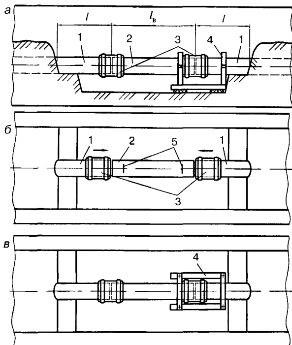
1 — концы газопровода, 2 — трубная вставка; 3 — муфты; 4 — позиционер для сборки соединения, 5 — метки установки муфт, l — длина освобождения концов газопровода; l_b — длина вставки
