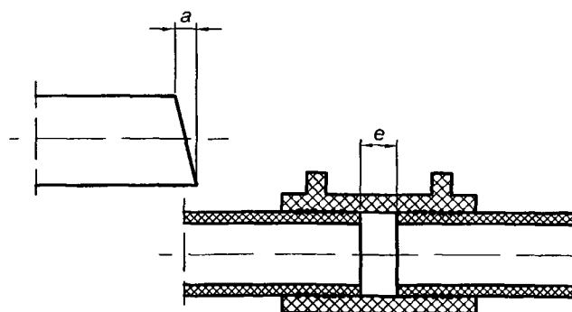
а — максимальный допуск косога среза трубы, е — максимальный зазор между двумя концами труб в муфте
