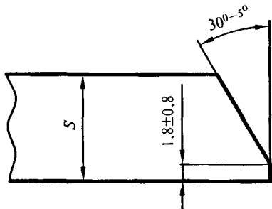
Рисунок 9 — Схема обработки кромок
