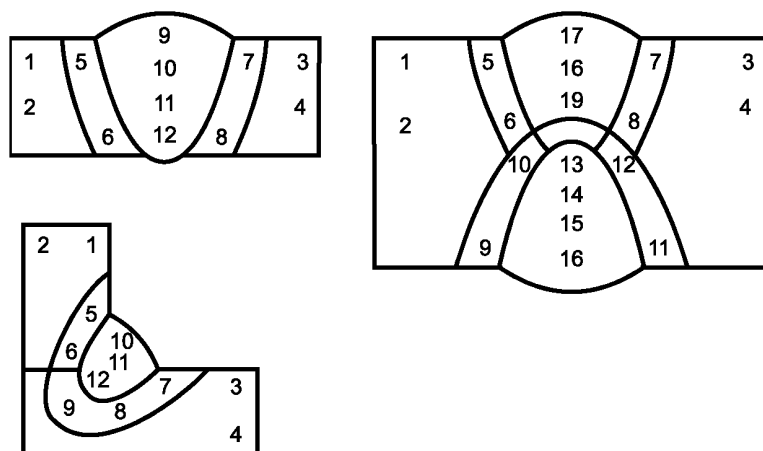
Участки замеров твердости (обозначены цифрами)
