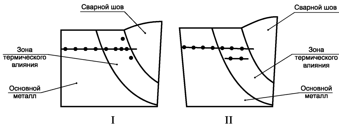
Схемы замеров твердости: I — основная, II — дополнительная
