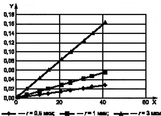
Рисунок А.1 — Интервал относительных удлинений согласно формуле (A.3)
